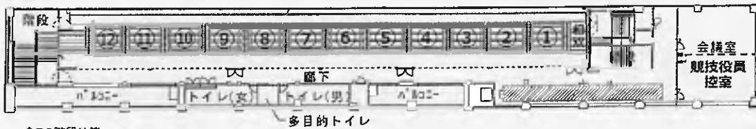
2階平面図
